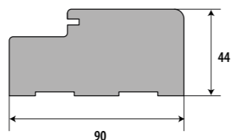
przekrój ościeznicy stałej
